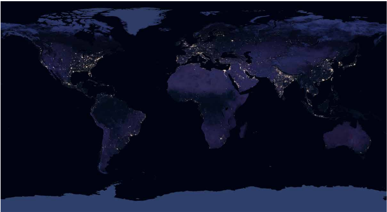
Die Erde bei Nacht, NASA/Noaa August 2017 | Foto: eoimages.gsfc.nasa.gov
